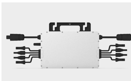
Mikro-Wechselrichter Hoymiles HM-1500
